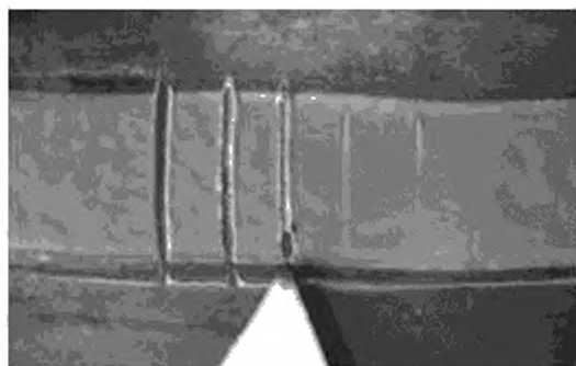
Рисунок А.4 – Оценка времени гелеобразования
