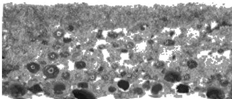
Рисунок A.10 – Максимально допустимая пористость поперечного сечения отслоенного покрытия
