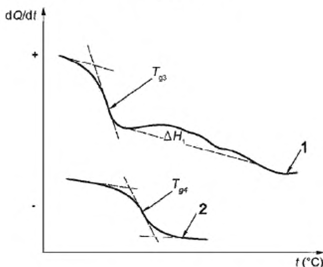
Рисунок A.6 – Примеры Термических диаграмм покрытия
