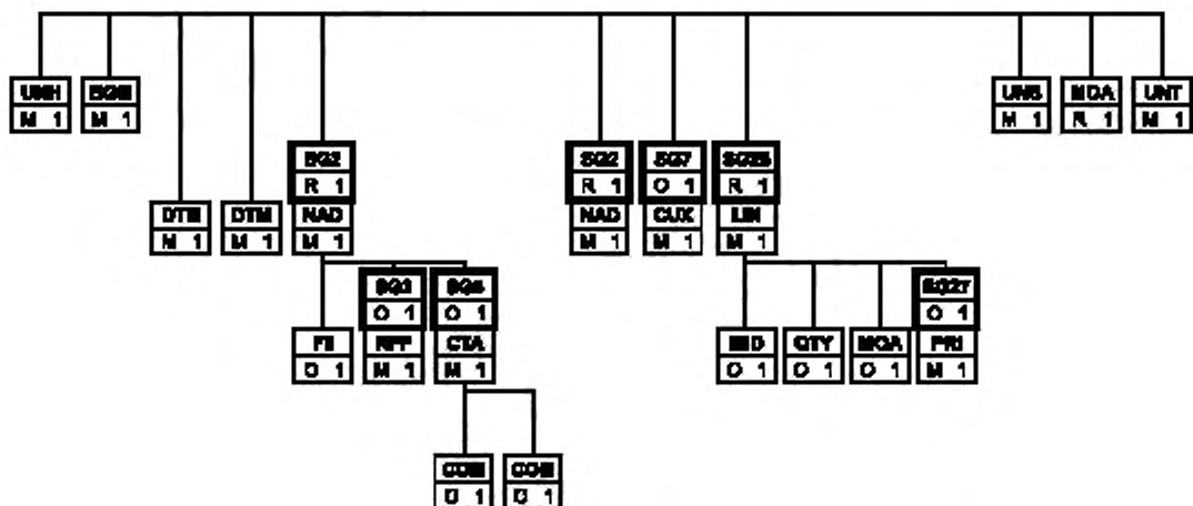
Рисунок A.1 — Диаграмма структуры сообщения (схема ветвления), основанная на EDIFACT ORDERS
