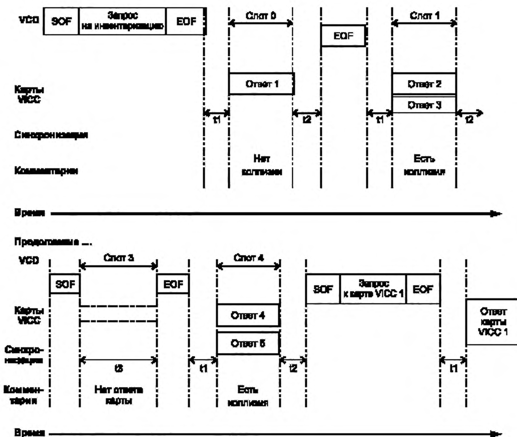
Рисунок 10 — Описание возможного алгоритма антиколлизии
