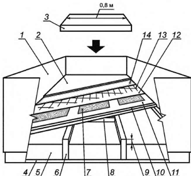
1 — деревянная доска; 2 — пол; 3 — кусок изоляции; 4 — опора для термоизоляции; 5 — термоизоляция; 6 — деревянный каркас 50 × 200 мм; 7 — нагревательный блок ; 8 — поперечный элемент; 9 — воздушный зазор (если предусмотрен); 10 — фанера; 11 — дополнительный материал (если предусмотрен); 12 — дополнительная электрическая изоляция (если предусмотрена); 13 — сетка; 14 — дополнительный слой (если предусмотрен)
