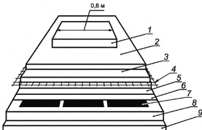
1 — кусок изоляции; 2 — пол; 3 — бетон; 4 — сетка (если предусмотрена); 5 — дополнительный слой (если предусмотрен); 6 — дополнительная электрическая изоляция (если предусмотрена); 7 — нагревательный блок ; 8 — термоизоляция; 9 — фанера
