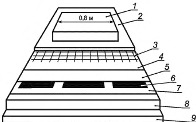
1 — кусок изоляции; 2 — пол; 3 — сетка; 4 — дополнительный слой (если предусмотрен); 5 — дополнительная электрическая изоляция (если предусмотрена); 6 — нагревательный блок ; 7 — дополнительный слой (если предусмотрен); 8 — термоизоляция; 9 — бетонное основание
