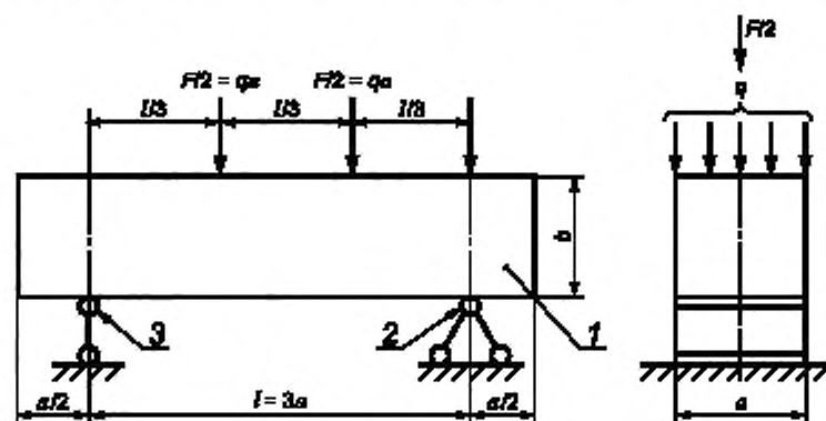
a — ширина и высота образца, F — нагрузка; q — распределенная нагрузка; l — пролет, 1 — образец; 2 — шарнирно-неподвижная опора; 3 — шарнирно-подвижная опора
