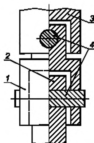
1 — центральный элемент; 2, 3 — концевые элементы; 4 — ось
