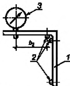
b_2 — база прибора; 1 — корпус (угольник), 2 — опора; 3 — индикатор
