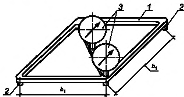
b_1 — база прибора; 1 — корпус (рамка); 2 — опора; 3 — индикатор
