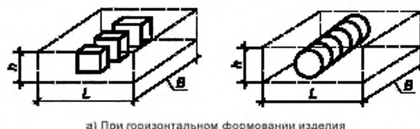
Рисунок 1 — Схемы выпиливания и выбурирования образцов ячеистого бетона (Лист 1)
