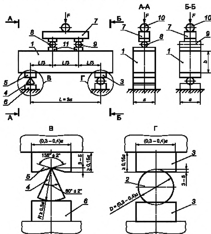
1 — образец; 2 — шар; 3 — опорная подушка; 4 — качающаяся призма; 5 — опорная сегментная подушка; 6 — опорная плоская подушка; 7 — распределительная траверса; 8 — шарнирно-неподвижная опора; 9 — шарнирно-подвижная опора; 10 — шаровой шарнир; 11 — стальная опорная пластина
