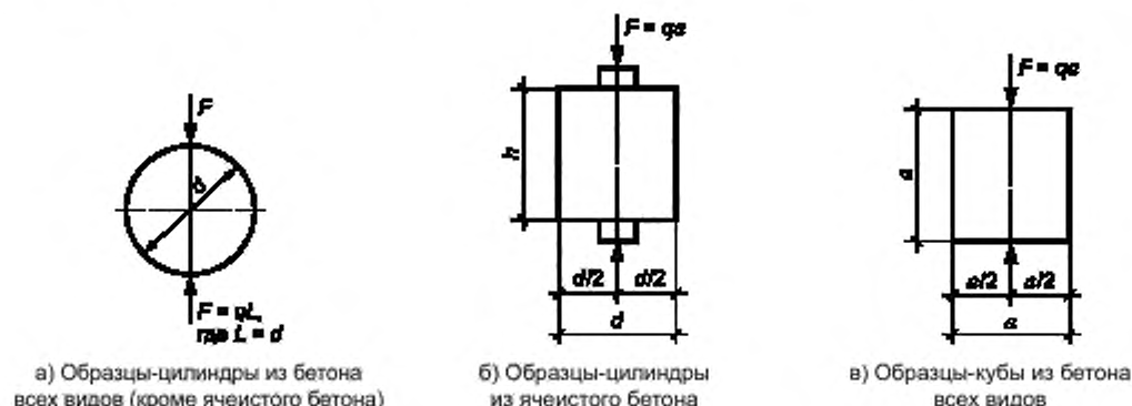
Рисунок 3 — Схемы испытания на растяжение при раскалывании (Лист 1)
