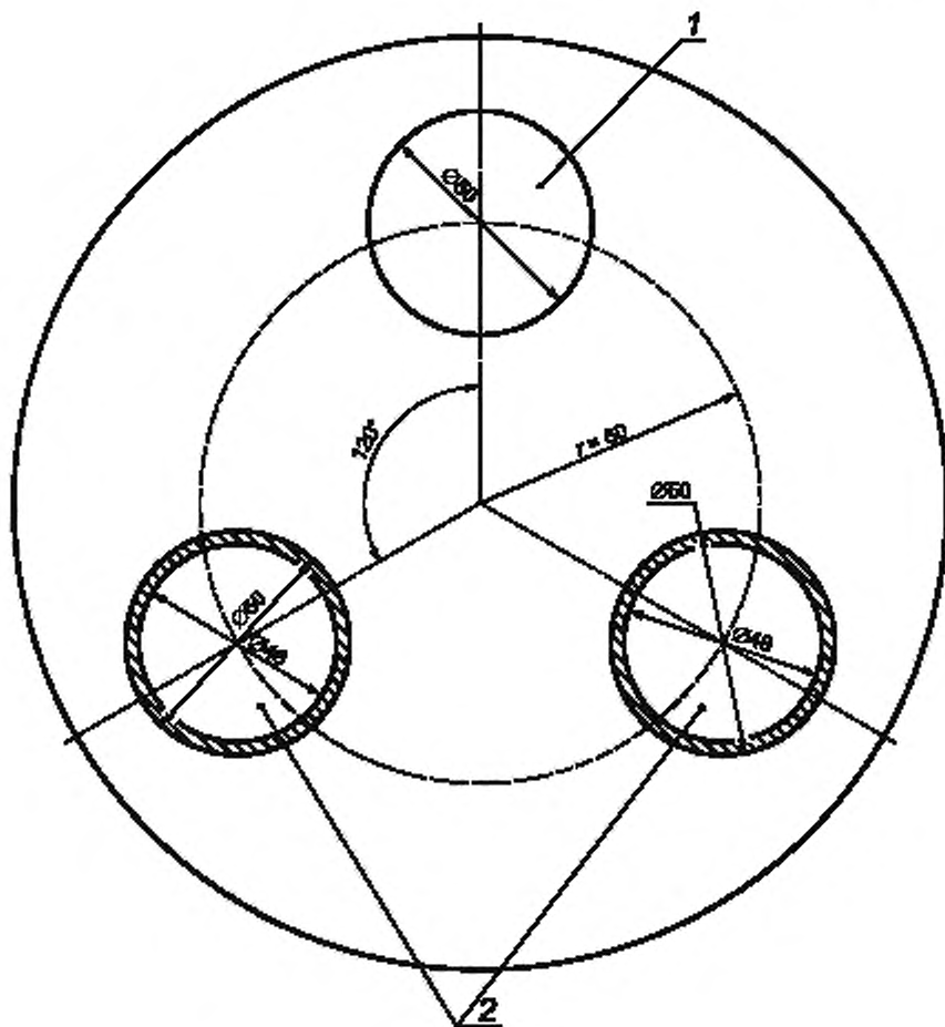
1 — твердый политетрафлюорэтилен; 2 — наполненные цилиндры
