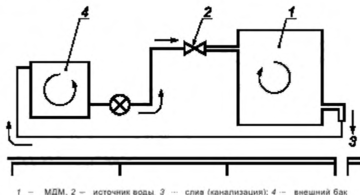
1 — МДМ, 2 — источник воды, 3 — слив (канализация); 4 — внешний бак
