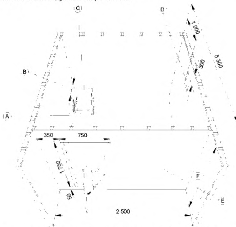
А – впуск воздуха; В – регулируемое расстояние; С – нагреватель для сауны; D – выпуск воздуха; E – передвижная стена; F – высота потолка 1900, 2100 или 2300 мм Рисунок АА.1 – Помещение сауны
