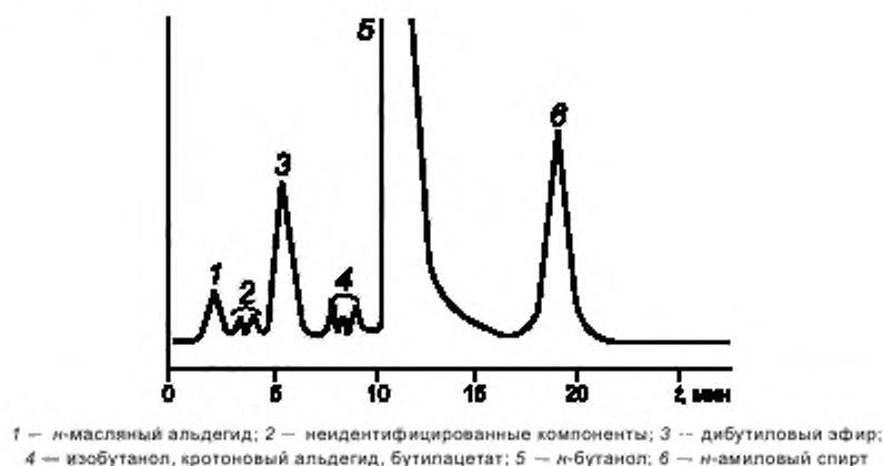
Рисунок 1 — Типовая хроматограмма n -бутанола, получаемого методом альдолиза ацетальдегида
