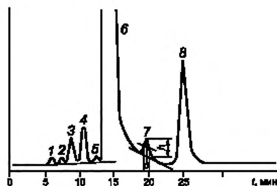
1 — дибутиловый эфир; 2 — n -бутилформат; 3, 5 — неидентифицированные компоненты; 4 — изобутанол; 6 — n -бутанол; 7 — изоамиловый спирт; 8 — n -амиловый спирт
