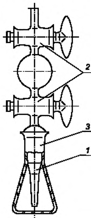
1 — пипетка; 2 — кран; 3 — колба с пришлифованным горлом
