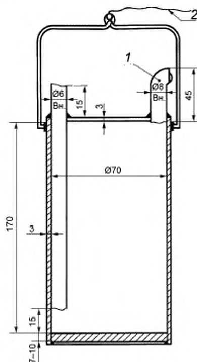
Рисунок 1 — Пробоотборник
