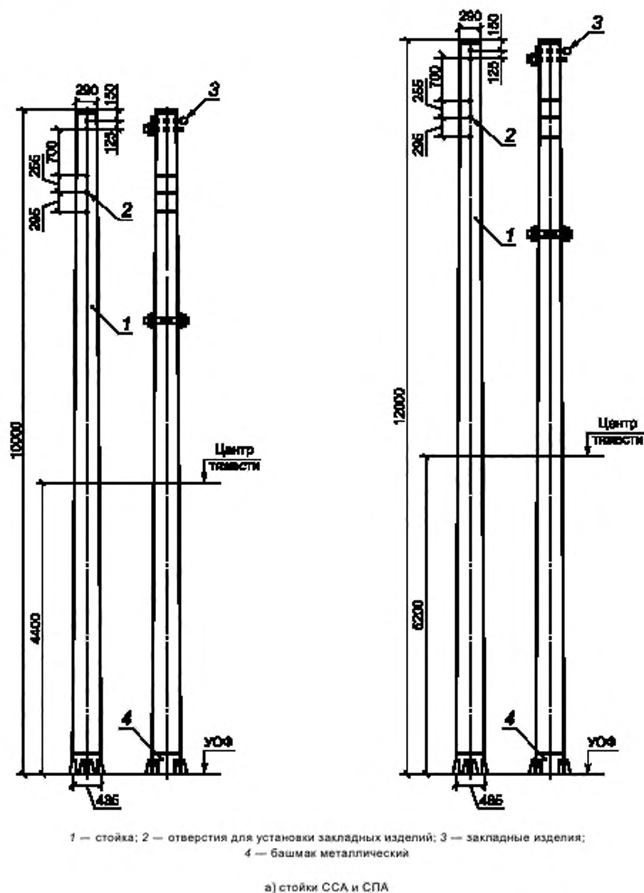
Рисунок А.2 — Стойки железобетонные 2-го типа по исполнению
