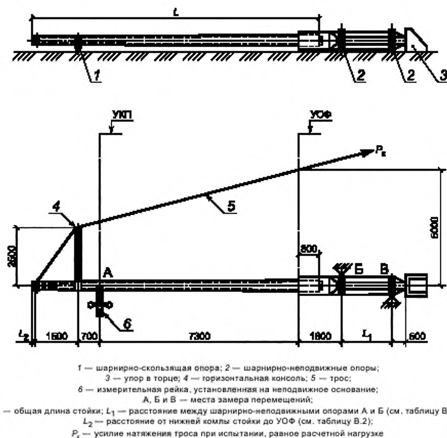
а) стойки СС и СП
