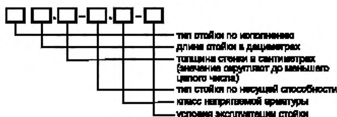
Рисунок Б.1 — Пример условного обозначения стоек железобетонных
