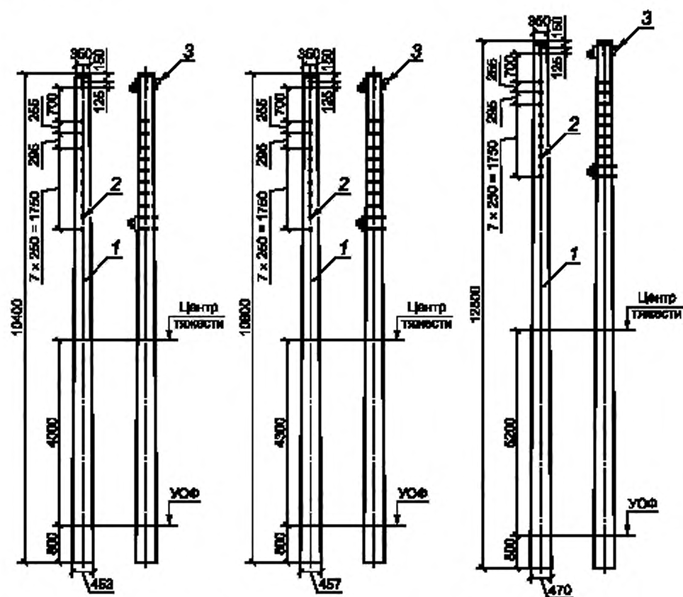
б) стойки СТ
