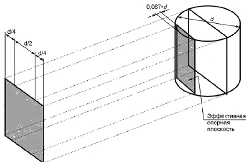
Рисунок 1 — Положение эффективной опорной плоскости для люксметра с цилиндрической и полусилиндрической насадками
