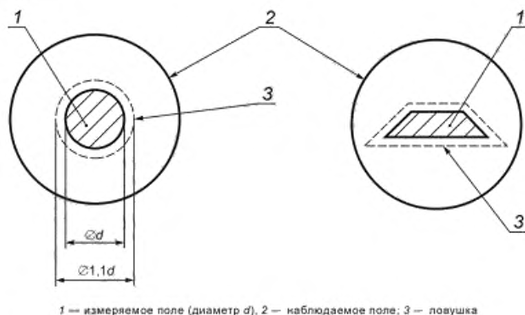
Рисунок 13 — Положение и размеры ловушки для измерений параметров функции f_{2,u}
