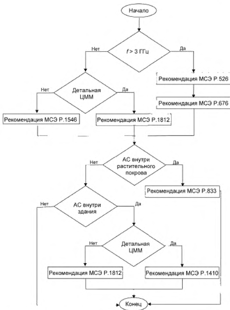
Рисунок 4.3 — Блок-схема алгоритма расчета ослабления радиосигнала на трассе
