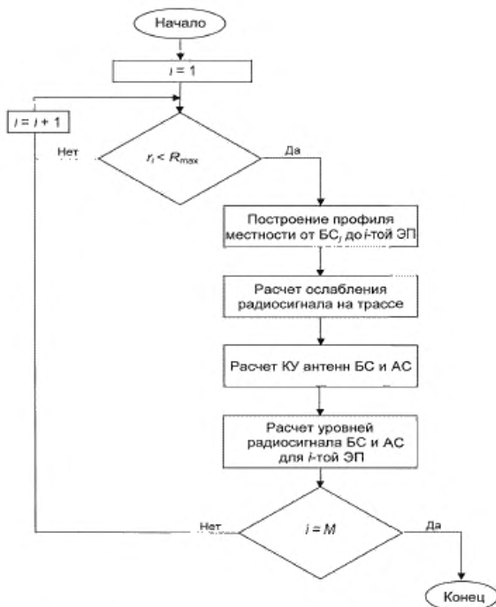
Рисунок 4.2 — Блок-схема алгоритма построения радиопокрытия БС
