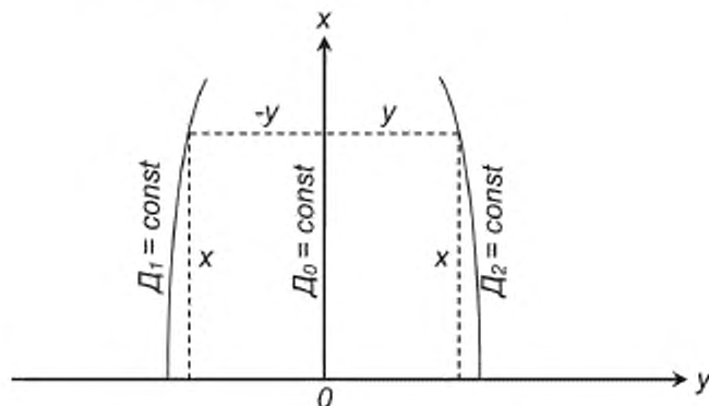
Рисунок А.1— Связь геодезических и плоских координат
