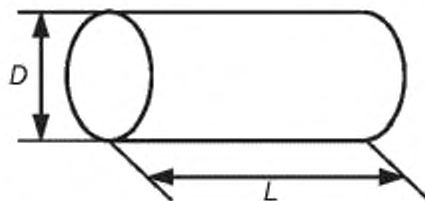
Рисунок 1 — Размеры пеллет
