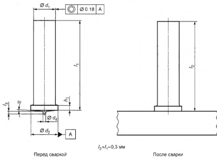
Рисунок 10 — Шпилька без резьбы (УТ)
