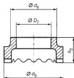
Рисунок 12 — Керамическое кольцо для шпильки с резьбой (PF)
