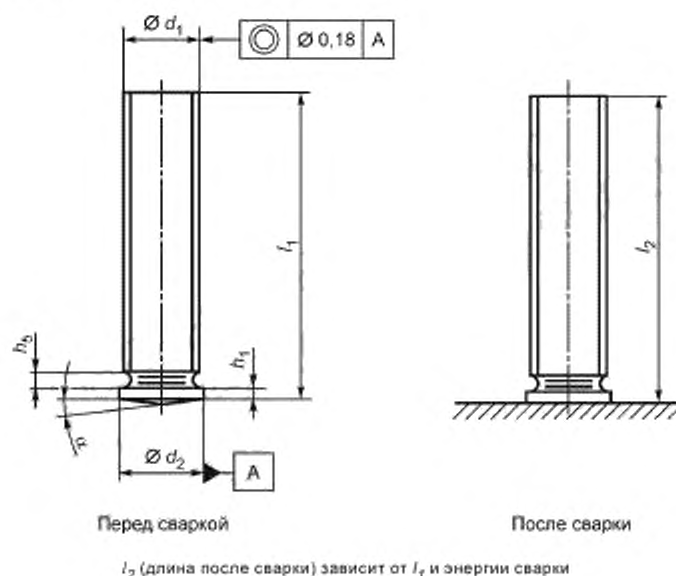
Рисунок 6 — Шпилька с резьбой с фланцем (PS)
