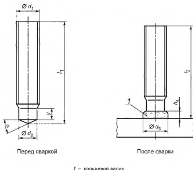
Рисунок 2 — Шпилька с резьбой с редуцированным стержнем (RD)
