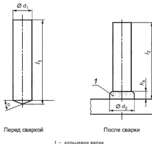
Рисунок 3 — Шпилька без резьбы (UD)
