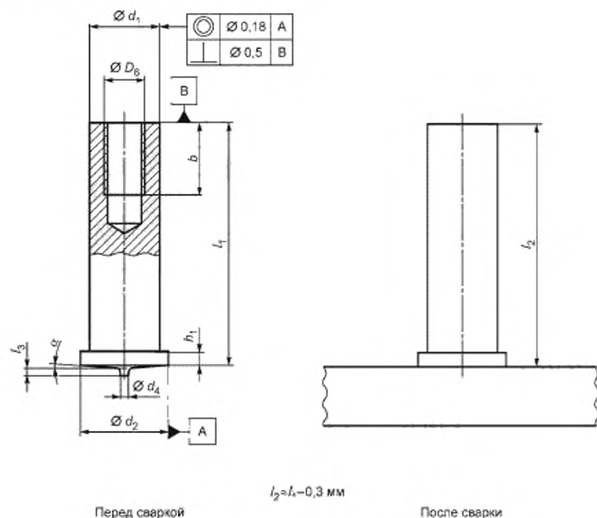
Рисунок 11 — Шпилька с внутренней резьбой (IT)
