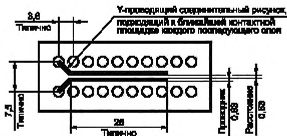
Рисунок В.6 — Тест-купон E
