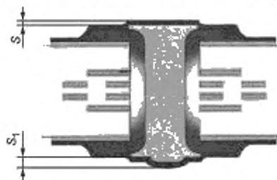
S — толщина крышки; S_1 — размер выступа крышки
