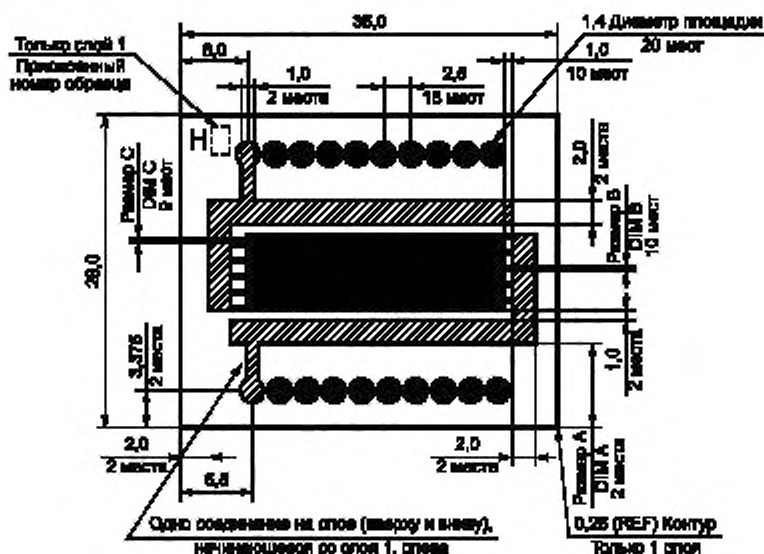
Рисунок В.7 — Тест-купон H
