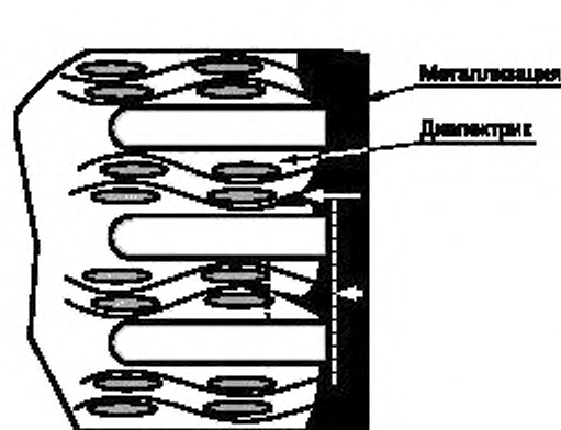
Рисунок 7 — Травление диэлектрика
