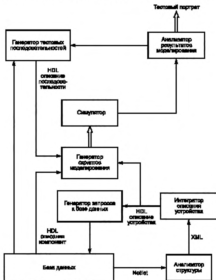
Рисунок 2 — Взаимосвязь компонентов системы автоматизированного построения тестов
