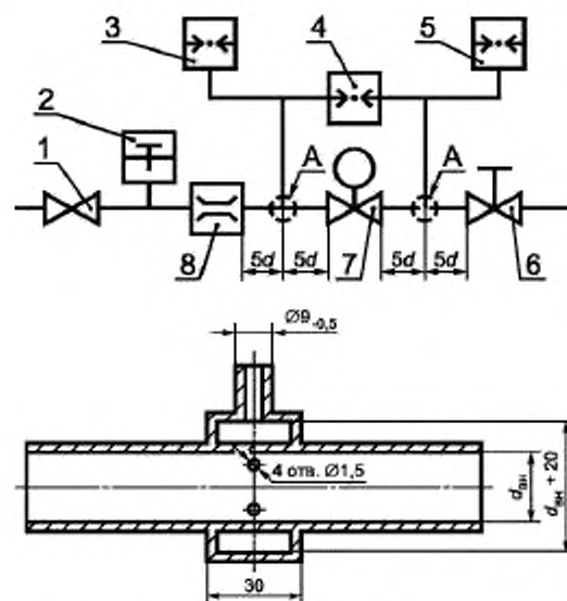
А — деталь; d_{вн} — внутренний диаметр трубки; d — наружный диаметр трубки; 1 — регулятор давления; 2 — термометр; 3, 5 — манометры; 4 — дифференциальный манометр; 6 — регулировочный кран; 7 — испытуемый образец; 8 — расходомер
