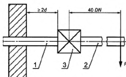
d – наружный диаметр; 1 – труба; 2 – труба; 3 – испытываемый образец
