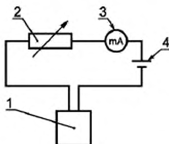
1 — испытуемый образец устройства контроля пламени; 2 — реостат; 3 — миллиампер; 4 — источник постоянного тока
