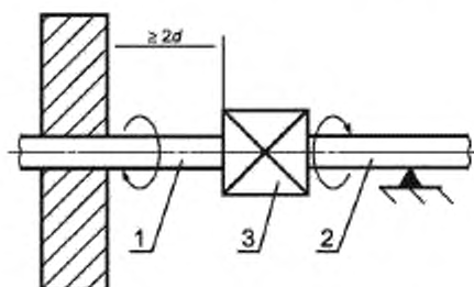
Рисунок 5 – Схема испытания устройства контроля пламени на кручение
