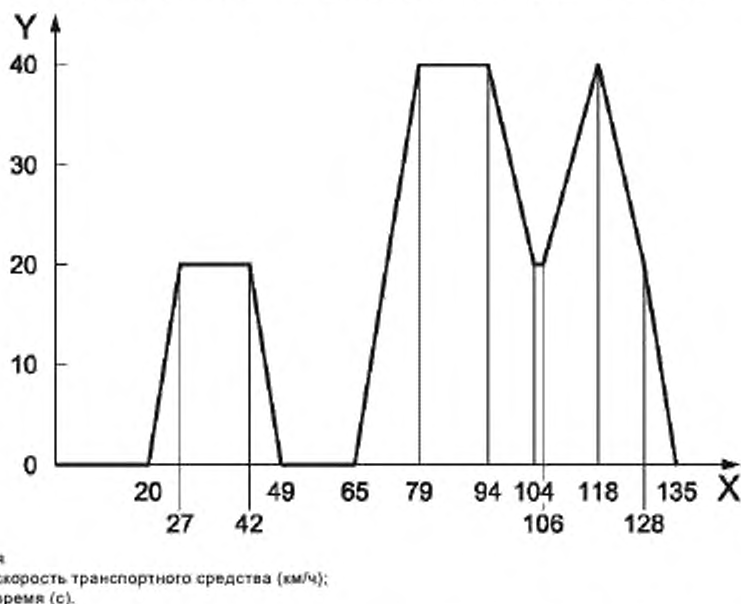
Рисунок А.1 — Последовательность испытаний транспортного средства по 10 режимному циклу
