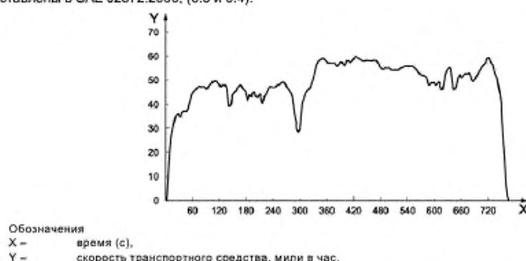
Рисунок С.2 — Последовательность испытаний транспортного средства, имитирующих загородное движение в условия США, в соответствии с загородным экономичным циклом движения (HFEDS)
