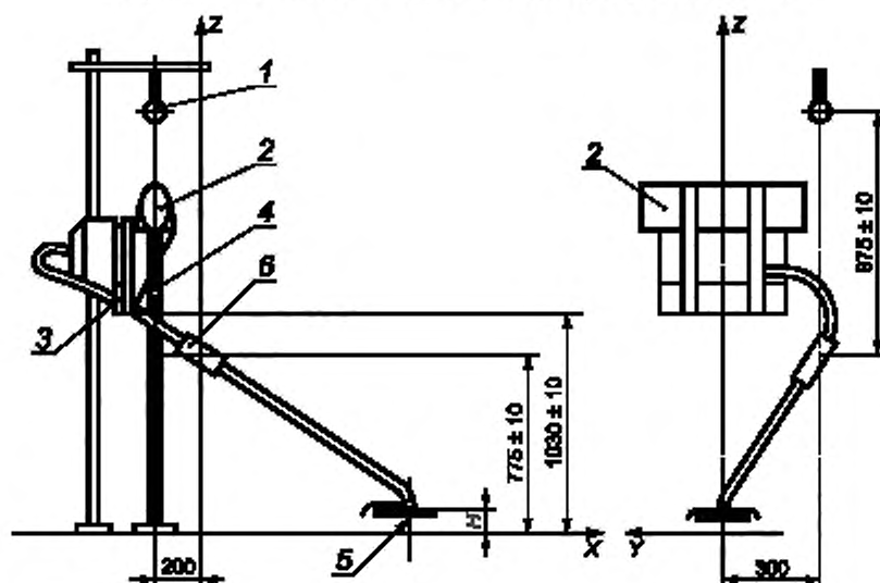
1 — микрофон (для измерений на рабочем месте оператора); 2 — устройство для крепления плечевых ремней; 3 — нижняя хромка ранца; 4 — устройство крепления машины; 5 — ось вращения режущего инструмента; 6 — задняя рукоятка
