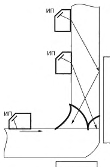
Рисунок 15 — Схема прозвучивания углового сварного соединения при одностороннем доступе совмещенными наклонными и прямыми преобразователями, преобразователями подповерхностных (головных) волн
