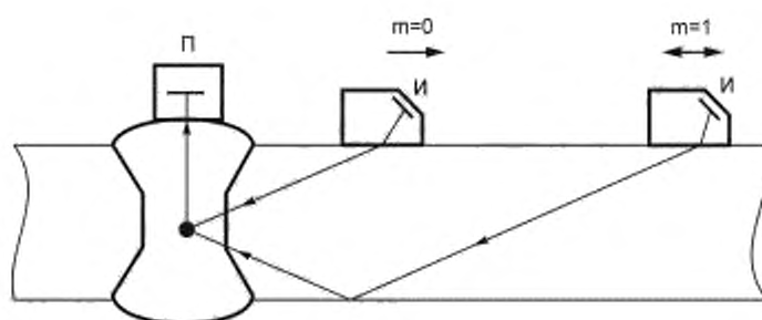
Рисунок 6 — Варианты дельта-метода
