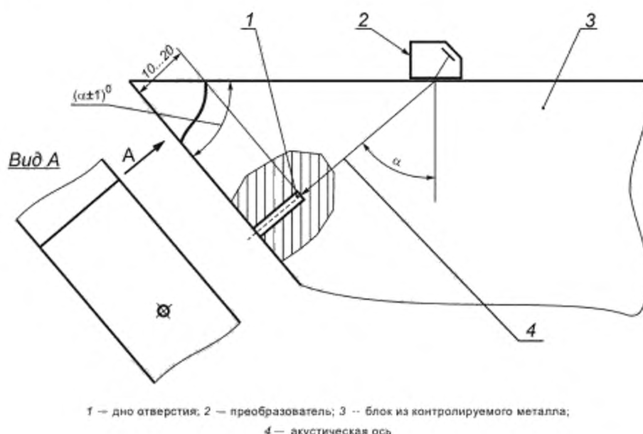
Рисунок Б.1 — Эскиз НО с плоскостным отражателем
