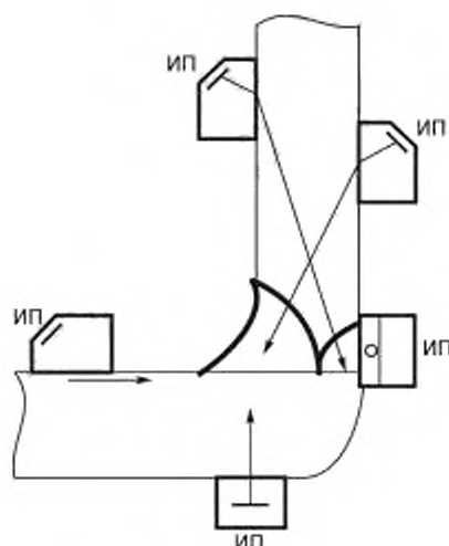
Рисунок 14 — Схема прозвучивания углового сварного соединения при двустороннем доступе совмещенными наклонными и прямым преобразователями, преобразователями поверхностных (головных) волн
