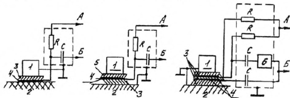
1 — проверяемые ПЭП; 2 — акустическая нагрузка; 3 — конденсаторная бумага СКОМ-ОВН толщиной 4 — 15 мкм или целлофановая пленка толщиной не более 22 мкм; 4 — алюминиевая фольга толщиной 5 — 1,2 мкм; 5 — лавсановая пленка ПЭТФ толщиной 10 — 15 мкм; 6 — фазоинвертор; 7 — резистор МЛТ-0,25 — 1 МОм; 8 — конденсатор К73-400 В-0,1 мкФ
