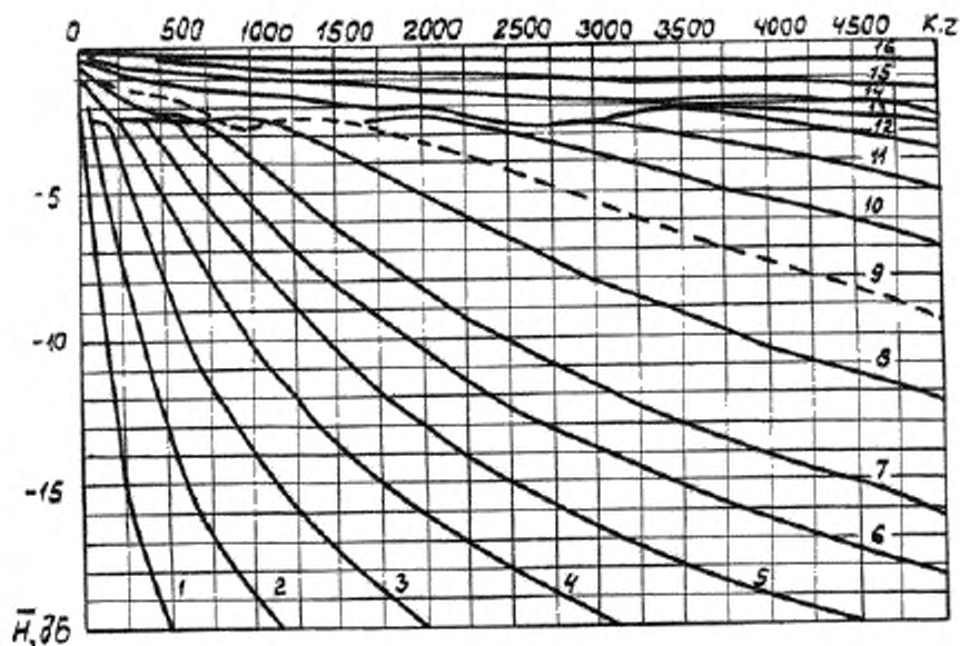
1 — ka = 10 ; 2 — ka = 15 ; 3 — ka = 20 ; 4 — ka = 25 ; 5 — ka = 30 ; 6 — ka = 35 ; 7 — ka = 40 ; 8 — ka = 50 ; 9 — ka = 60 ; 10 — ka = 70 ; 11 — ka = 80 ; 12 — ka = 90 ; 13 — ka = 100 ; 14 — ka = 150 ; 15 — ka = 160 — 400; 17 — ka = 500 — 1600
