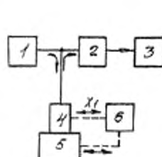
1 — генератор радиопульсов; 2 — приемник; 3 — осциллограф; 4 — проверяемый ПЭП; 5 — акустическая нагрузка; 6 — устройство ориентации
