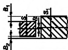
Рисунок 15 — Смещение кромок
