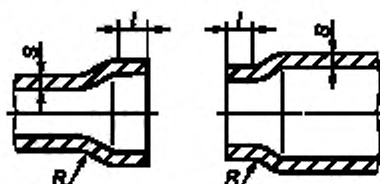
Рисунок 5 — Отбортованный и переходный элемент
