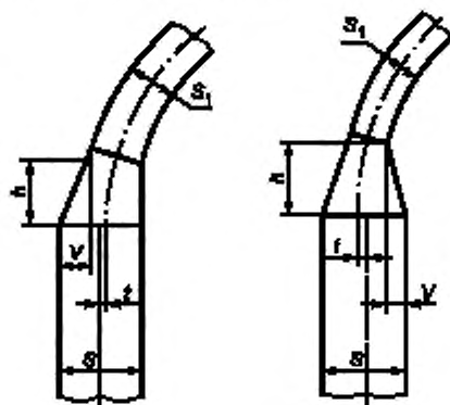
Рисунок 2 — Узел соединения днища с обечайкой
