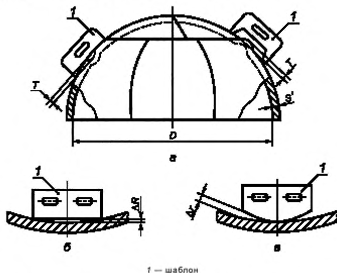
Рисунок 7 — Отклонение формы полусферического днища
