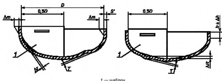
Рисунок 6 — Отклонение размеров и формы эллиптического днища
