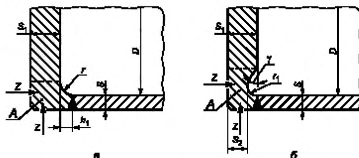
Рисунок 4 — Плоские днища
