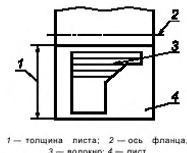
Рисунок 8 — Схема вальцовки фланца приварного встык по плоскости листа
