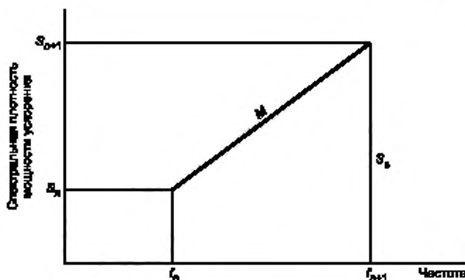
Рисунок А.5 — График спектральной плотности ускорения в полосе частот
