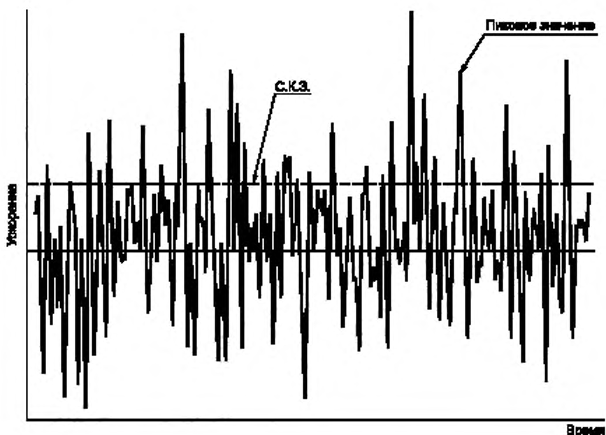
Рисунок А.2 — Отсечка (ограничение) сигнала
