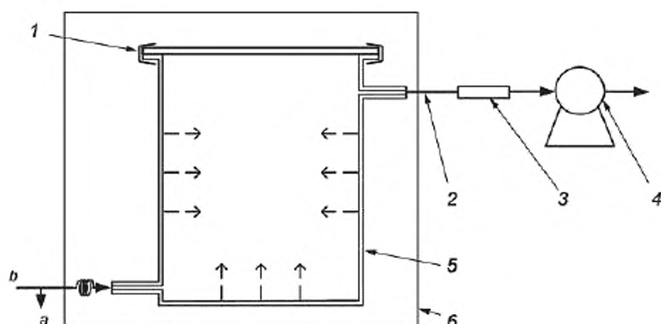
1 – зажим; 2 – линия передачи; 3 – сорбционная трубка; 4 – побудитель расхода; 5 – микрокамера; 6 – устройство нагрева камеры (до температуры 200 °С – 220 °С); а – линия сброса избытка газа; б – линия подачи инертного газа (He или N 2 )
