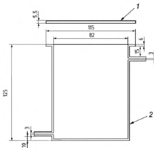
1 – крышка; 2 – контейнер
