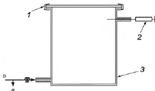
1 – зажим; 2 – микрошприц; 3 – микрокамера; а – линия сброса избытка газа; b – линия подачи инертного газа (He или N 2 )
