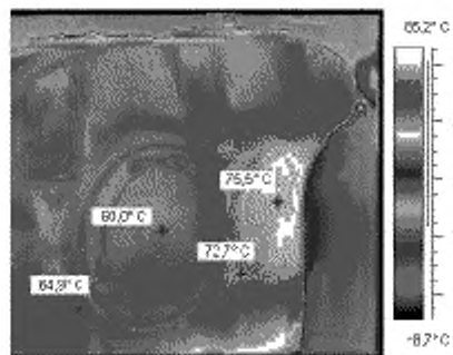
Рисунок С.5 – Редуктор со стороны двигателя
