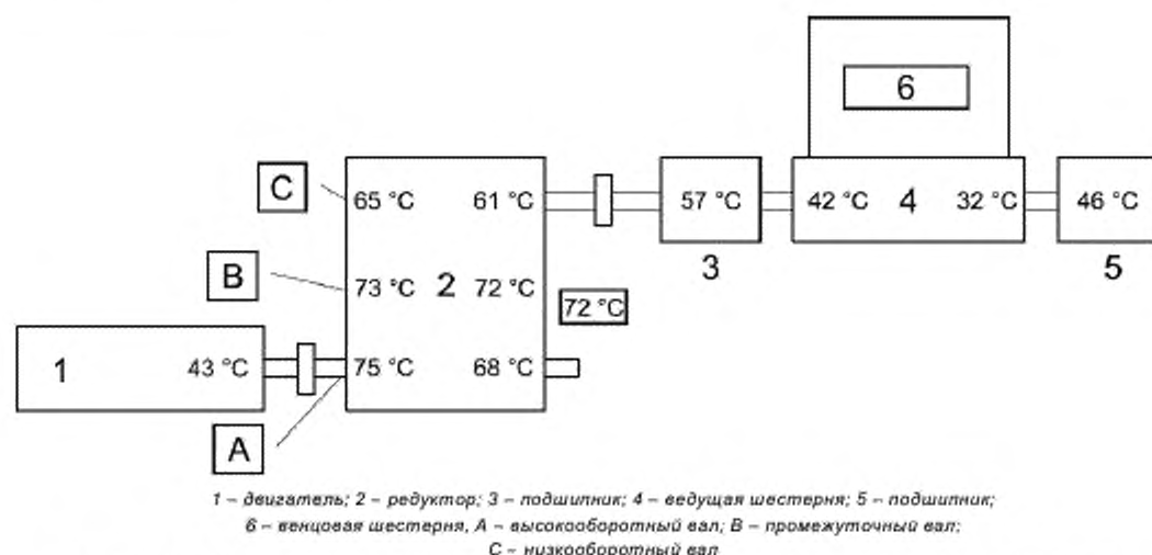
Рисунок С.2 – Результаты измерений температуры на схеме механизма привода шаровой мельницы
