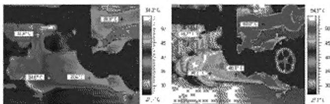
Рисунок С.10 – Термограммы двух маслоохладителей
