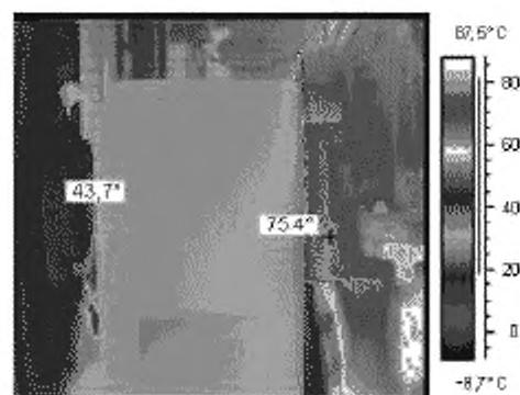
Рисунок С.3 – Двигатель и входной вал редуктора
