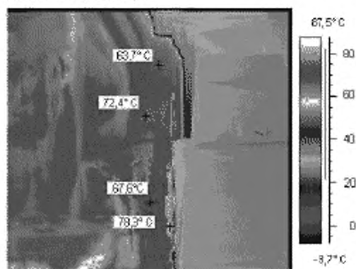
Рисунок С.4 – Редуктор со стороны входного вала
