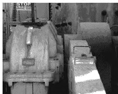
Рисунок С.4 – Редуктор со стороны входного вала
