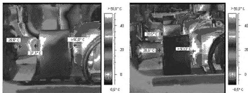
Рисунок С.9 – Термограммы насосов
