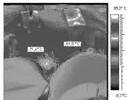
Рисунок С.6 – Редуктор со стороны мельницы
