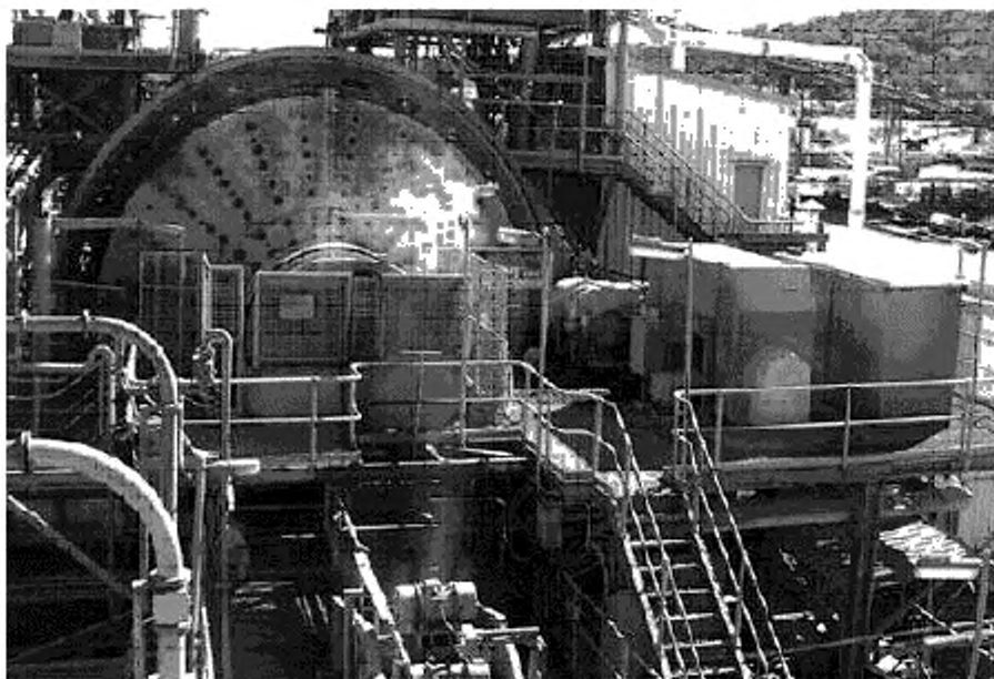
Рисунок С.1 – Рудоразмольная шаровая мельница с механизмом привода
