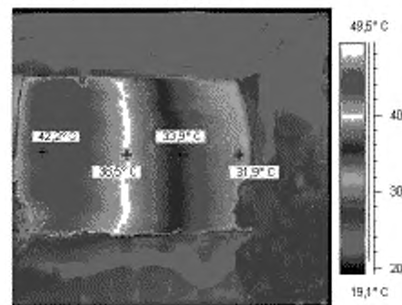
Рисунок С.8 – Ведущая шестерня привода мельницы
