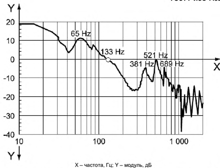
Рисунок В.2 – Диаграмма Бode типичной передаточной функции разомкнутой цепи G_o
