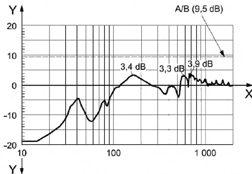
X – частота, Гц; Y – модуль, дБ; A/B – граница между зонами устойчивости (см. таблицу 1)
