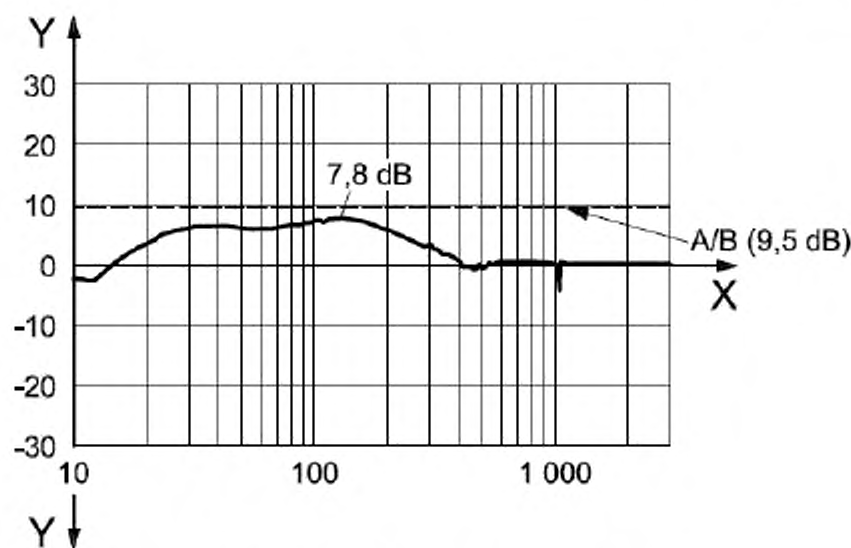
Рисунок С.3 – Функция чувствительности G_s ротора NEDO
