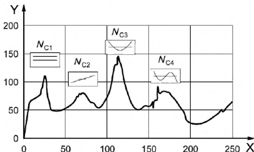
Рисунок A.10 – Изменение вибрации с изменением частоты вращения ротора
