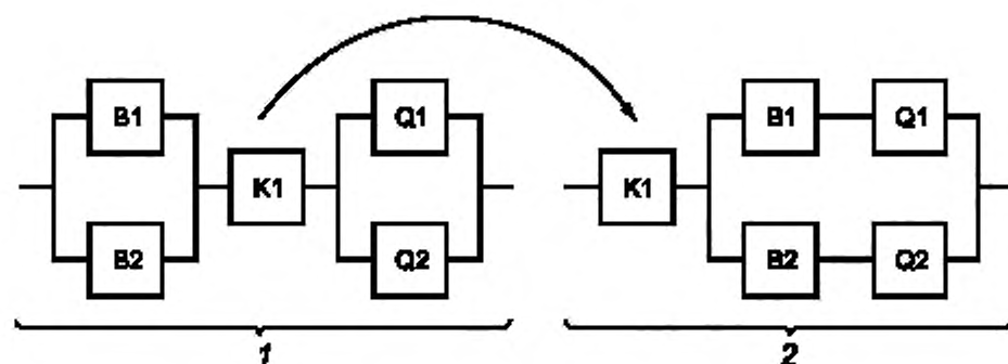
1 — Представление аппаратных средств: три подсистемы на уровне СБЗ/СУ; 2 — Упрощенное логическое представление: две подсистемы на уровне СБЗ/СУ
