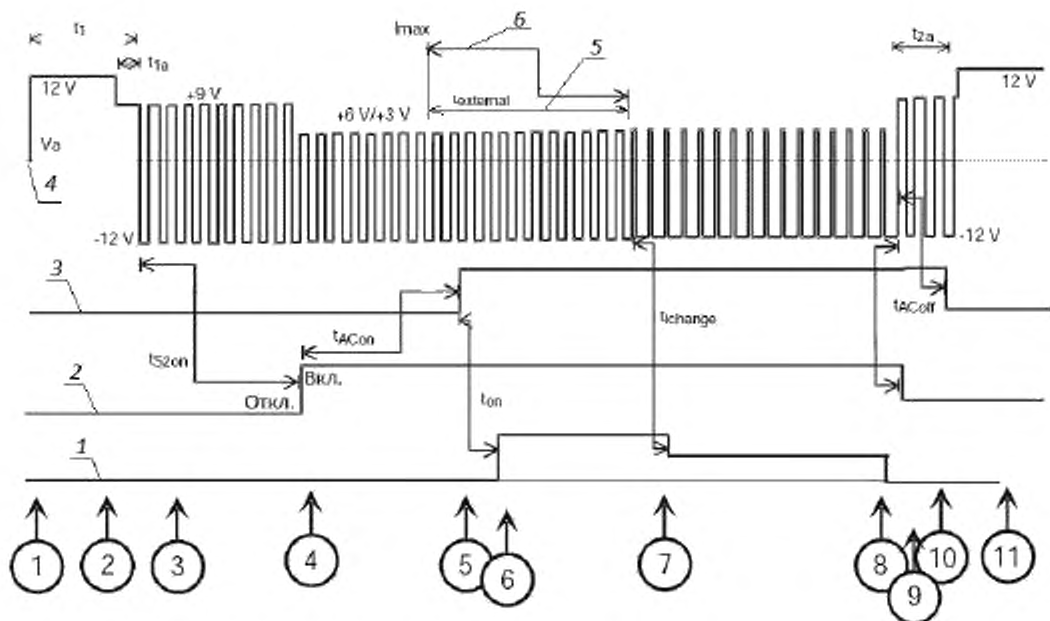
1 — подача переменного тока; 2 — состояние переключателя S2 ЭТ; 3 — напряжение питания переменного тока от точки; 4 — напряжение на контрольном проводе управления относительно земли; 5 — время вне контроля ОИПЭТ; 6 — команда подачи I_{max} .
