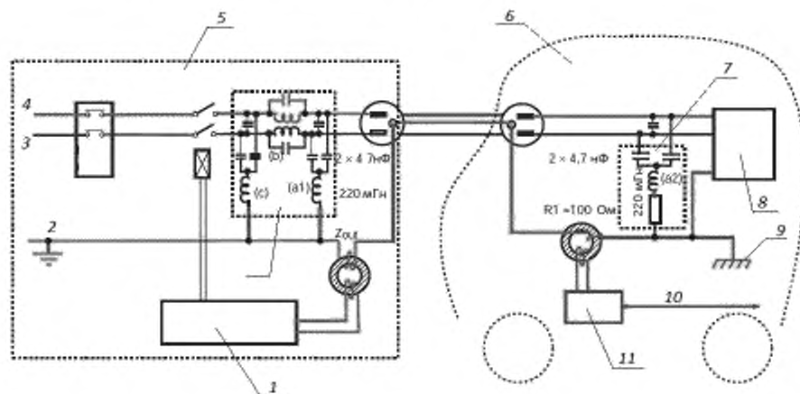
1 — модем с командным реле; 2 — земля; 3 — фильтр; 4 — нейтраль; 5 — стационарная силовая розетка; 6 — ЭТ или ПГДЭТ; 7 — ВЧ фильтр; 8 — зарядное устройство ЭТ; 9 — шасси ЭТ; 10 — команда ЭТ; 11 — модем
