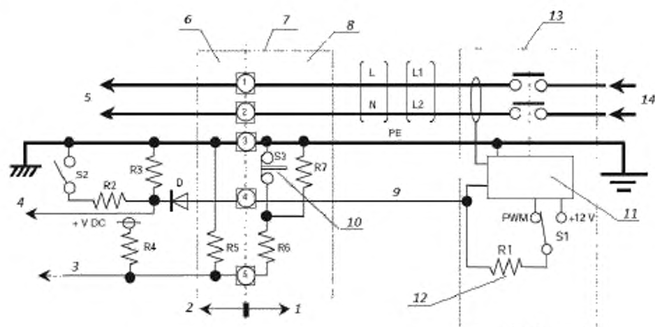
1 — комплект шнура; 2 — ЭТ; 3 — логическая схема обнаружения соединения; 4 — логическая схема функции контрольного управления; 5 — ввод зарядного устройства; 6 — ввод; 7 — соединитель ЭТ; 8 — переносная розетка; 9 — контрольное управление (провод контрольного управления); 10 — нажимной выключатель (нормально включен); 11 — контроллер функции контрольного управления; 12 — УДТ с функцией контрольного управления для замыкания цепи; 13 — силовое оборудование питания (зарядная станция); 14 — установка питания
