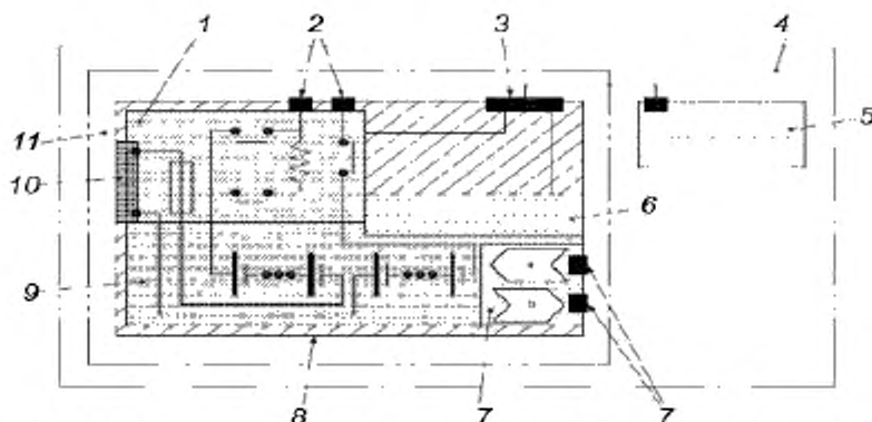
1 – электрические цепи напряжения класса В (соединители, предохранители, провода); 2 – выводы напряжения класса В; 3 – выводы напряжения класса А; 4 – батарейная система; 5 – BCU; 6 – электронная система аккумуляторов; 7 – система охлаждения и выводы системы охлаждения (в отдельных случаях); 8 – ударопрочный (для обычных условий применения) корпус; 9 – аккумуляторная подборка (аккумуляторы, датчики, элементы системы охлаждения); 10 – сервисное устройство отключения; 11 – батарейный блок; а – вход; б – выход
