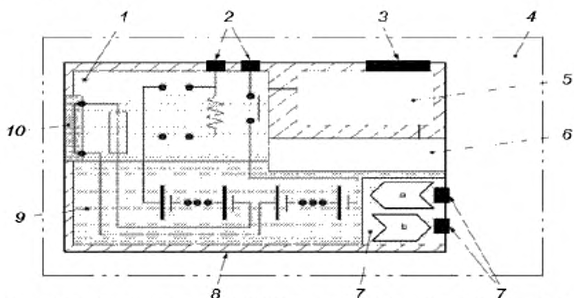
1 – электрические цепи напряжения класса В (соединители, предохранители, провода); 2 – выводы напряжения класса В; 3 – выводы напряжения класса А; 4 – батарейная система; 5 – BCU; 6 – электронная система аккумуляторов; 7 – система охлаждения и выводы системы охлаждения (в отдельных случаях); 8 – ударопрочный (для обычных условий применения) корпус; 9 – аккумуляторная подборка (аккумуляторы, датчики, элементы системы охлаждения); 10 – сервисное устройство отключения; а – вход; б – выход
