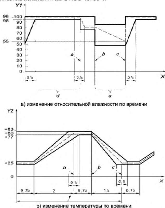
а) изменение относительной влажности по времени
