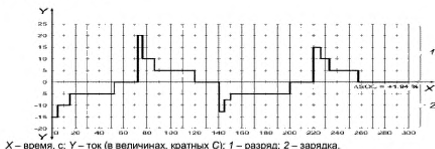
Рисунок 8 — Режим по току для циклического испытания на долговечность. Режим постепенной зарядки. Т а б л и ц а 18 — Изменение тока по времени в режиме постепенной зарядки
