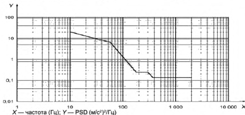
Рисунок 12 — Распределение PSD по частоте колебаний
