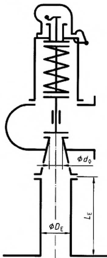
Рисунок 4.1 – Предохранительные клапаны
