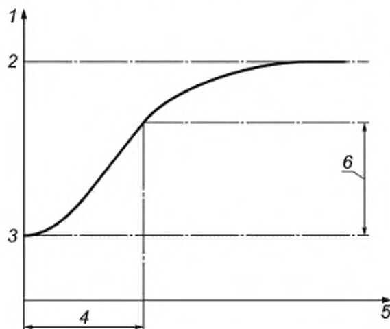
1 — t_n - t_a ; 2 — (t_n - t_a)_2 ; 3 — (t_n - t_a)_0 ; 4 — \tau_c ; 5 — Время; 6 — 0,632 ((t_n - t_a)_2 - (t_n - t_a)_0)
