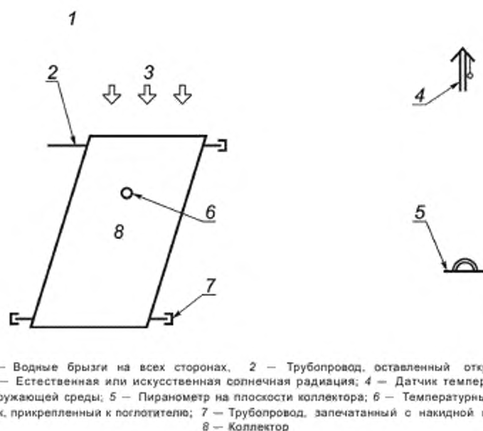
Рисунок А.8 — Описание схемы для испытания на внешний тепловой удар
