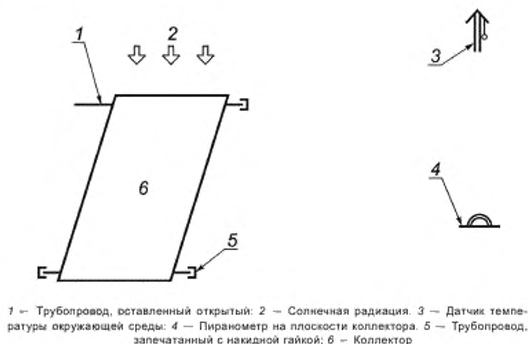
Рисунок А.7 — Описание схемы для испытания на воздействие атмосферных условий
