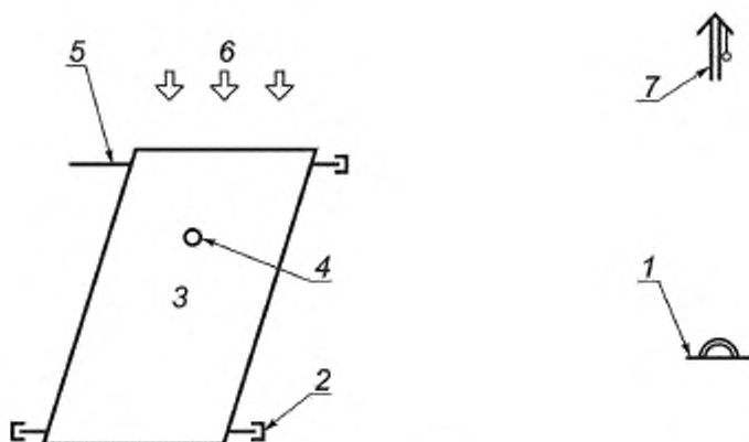
1 — Пирометр на плоскости коллектора; 2 — Трубопровод, запечатанный с накидной гайкой; 3 — Коллектор; 4 — Температурный датчик, прикрепленный к поглотителю; 5 — Трубопровод, оставленный открытым; 6 — Естественное или искусственное солнечное излучение; 7 — Датчик температуры окружающей среды
