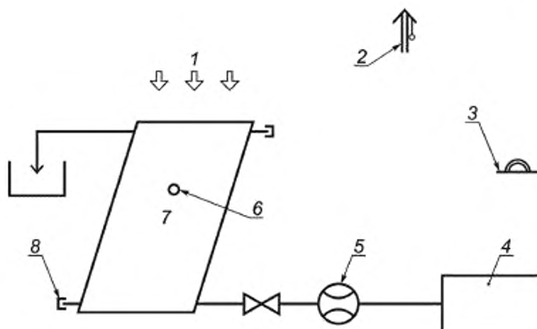
1 — Естественная или искусственная солнечная радиация; 2 — Датчик температуры окружающей среды; 3 — Пирометр на плоскости коллектора; 4 — Источник жидкости теплоносителя; 5 — Расходомер; 6 — Температурный датчик, прикрепленный к поглотителю; 7 — Коллектор; 8 — Трубопровод, запечатанный с накидной гайкой
