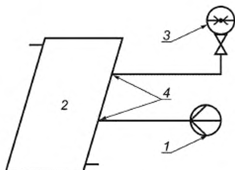
1 — Источник пневматического давления; 2 — Коллектор; 3 — Манометр; 4 — Отверстия в зазоре между покрытием коллектора и поглотителем
