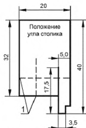
Рисунок 1 – Форма и размер образца для испытания
