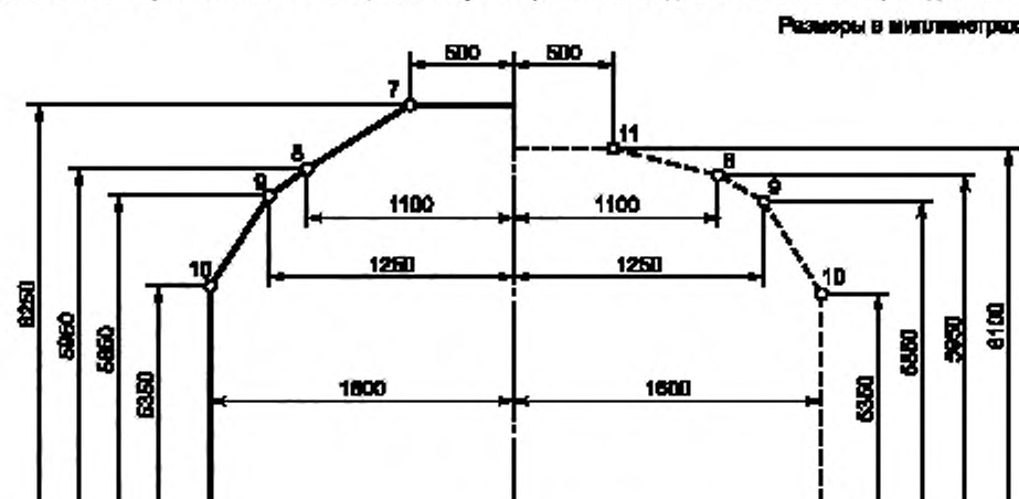
Рисунок В.2 — Минимальное очертание верхней части сооружений при напряжении в контактной сети (1,5—4) кВ
