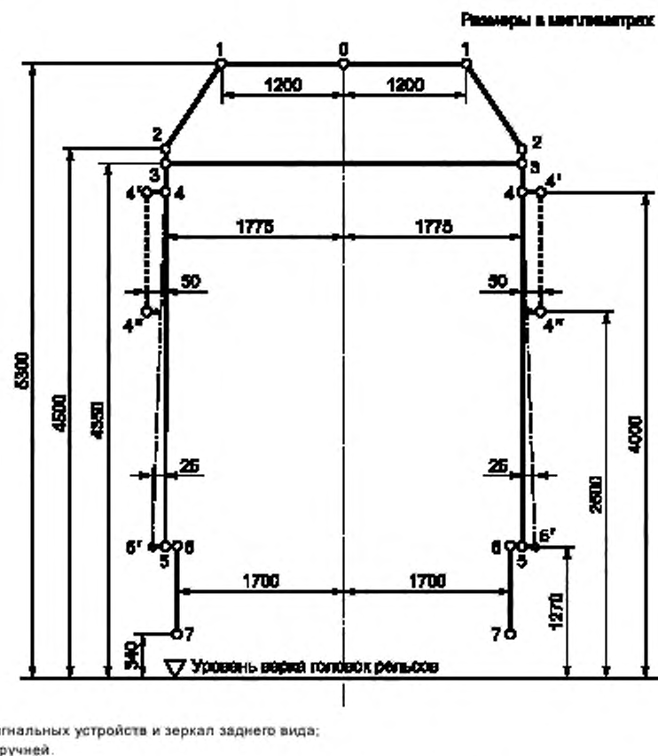
Рисунок 3 — Статический габарит T_{лр}
