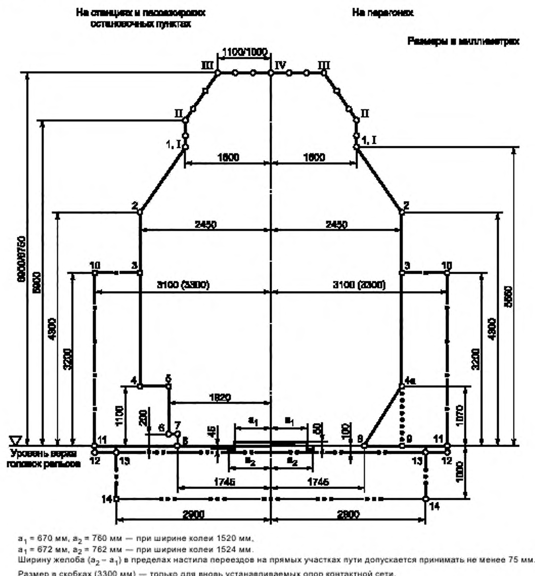
Рисунок 26 — Габарит C_{750}
