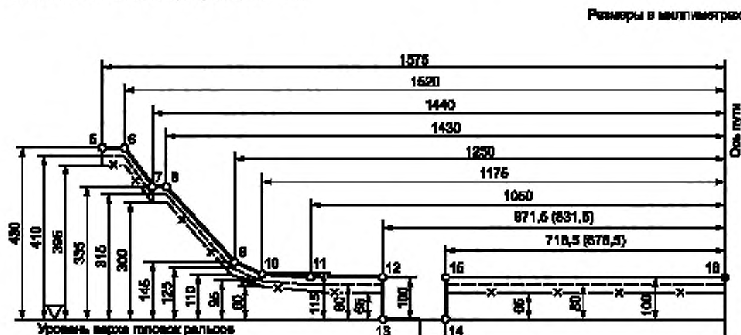
Рисунок 20 — Нижнее очертание габарита для подвижного состава, не проходящего сортировочные горки, оборудованные вагонными замедлителями
