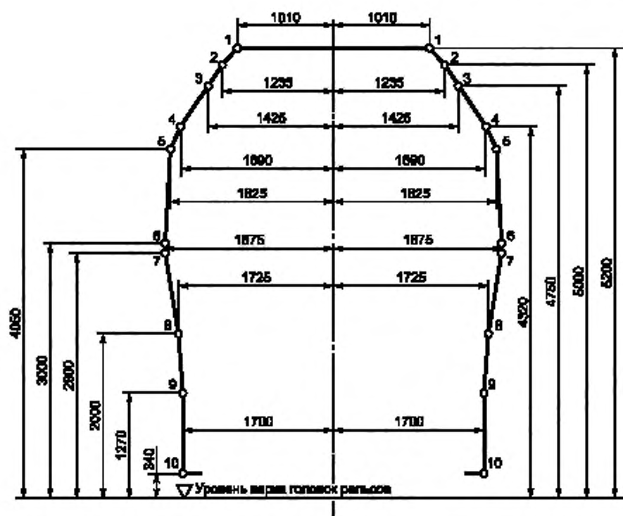
Рисунок 2 — Статический габарит T_{\text{ц}}
