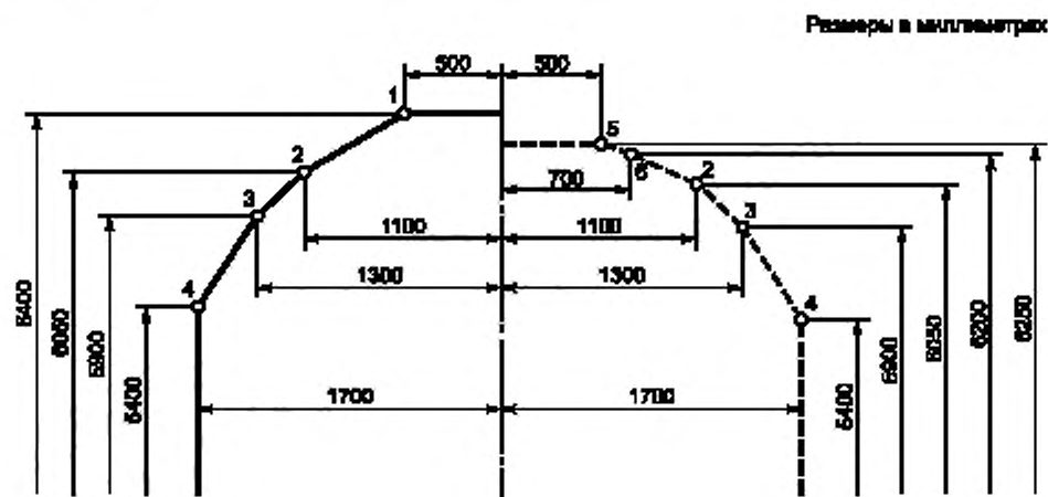
Рисунок В.1 — Минимальное очертание верхней части сооружений при напряжении в контактной сети 25 кВ
