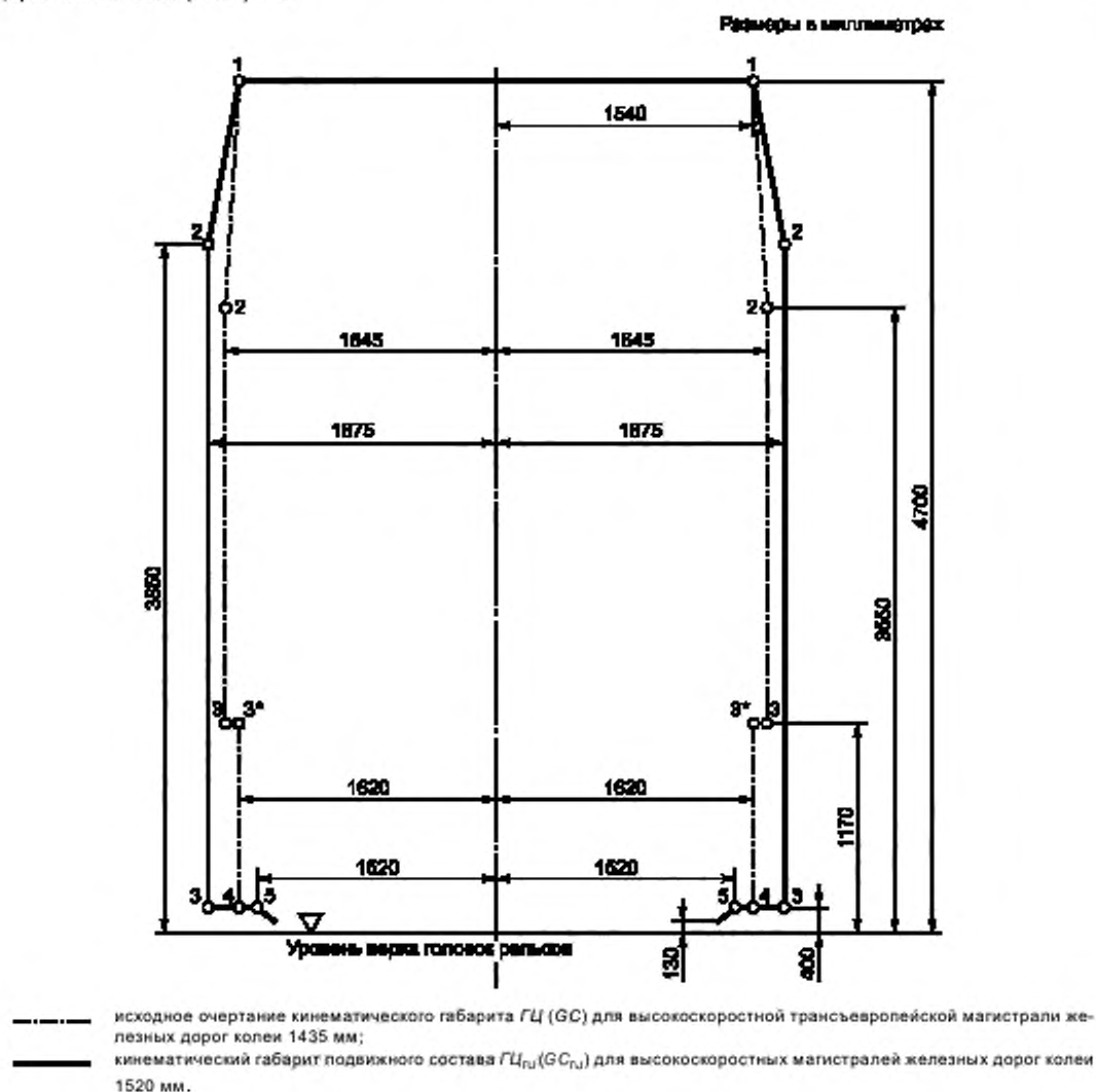
Рисунок 9 — Габарит подвижного состава ГЦ ( GC ) и гармонизированный с ним габарит ГЦ_{гу} ( GC_{гу} )
