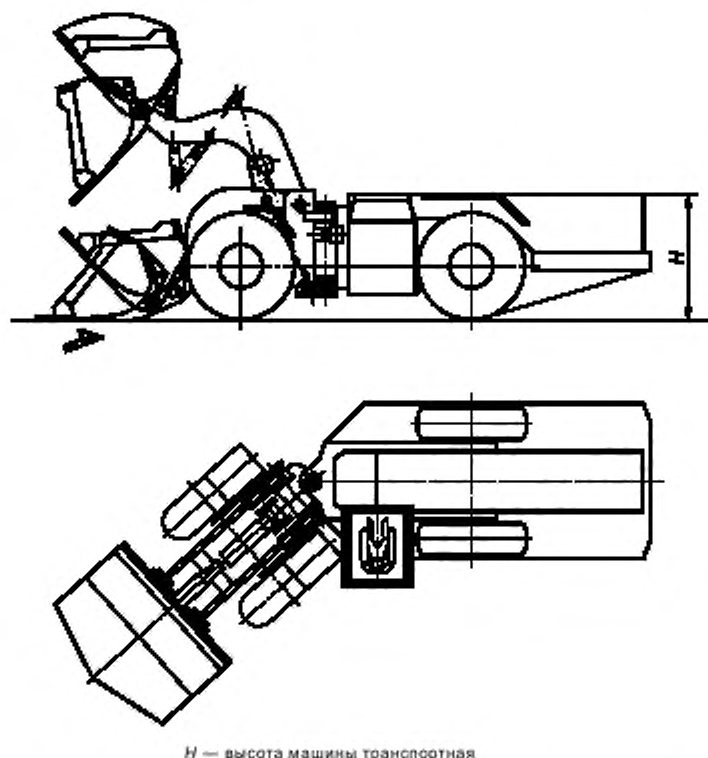
Рисунок 3 — Машина низкопрофильная с кабиной машиниста, вынесенной относительно продольной оси
