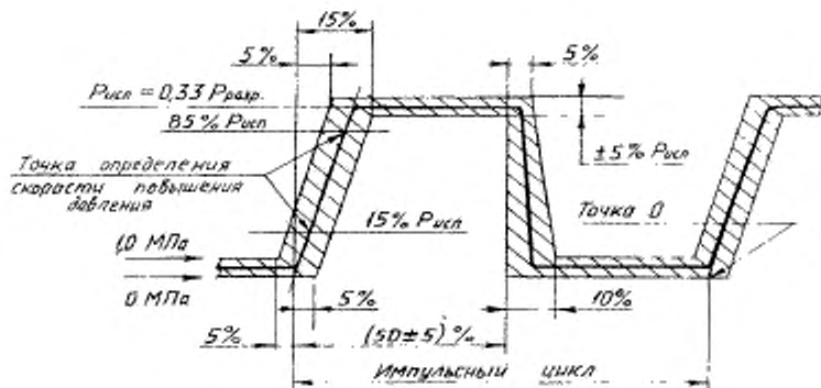
Рисунок 1 – Импульсный цикл динамических испытаний рукавов
