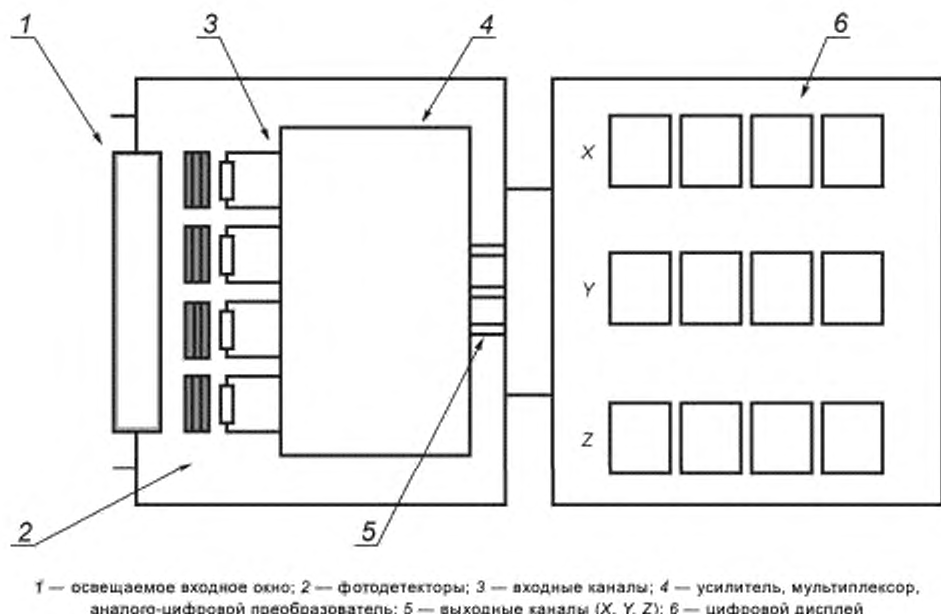
Рисунок 1 — Схематическое изображение колориметра
