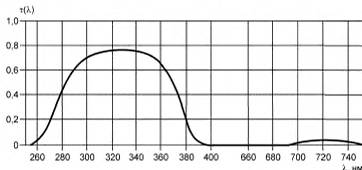
Рисунок 3 — Спектральный коэффициент пропускания \tau(\lambda) корректирующего УФ-фильтра
