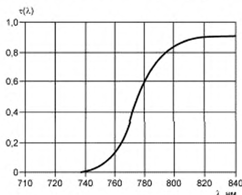
Рисунок 4 — Спектральный коэффициент пропускания \tau(\lambda) корректирующего ИК-фильтра
