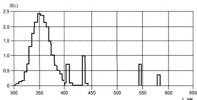
Рисунок 2 — Спектральное распределение излучения лампы
