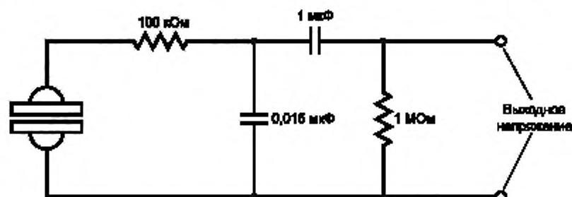
Рисунок 201.109 — Испытательный контур для определения нестабильности смещения/внутреннего шума
