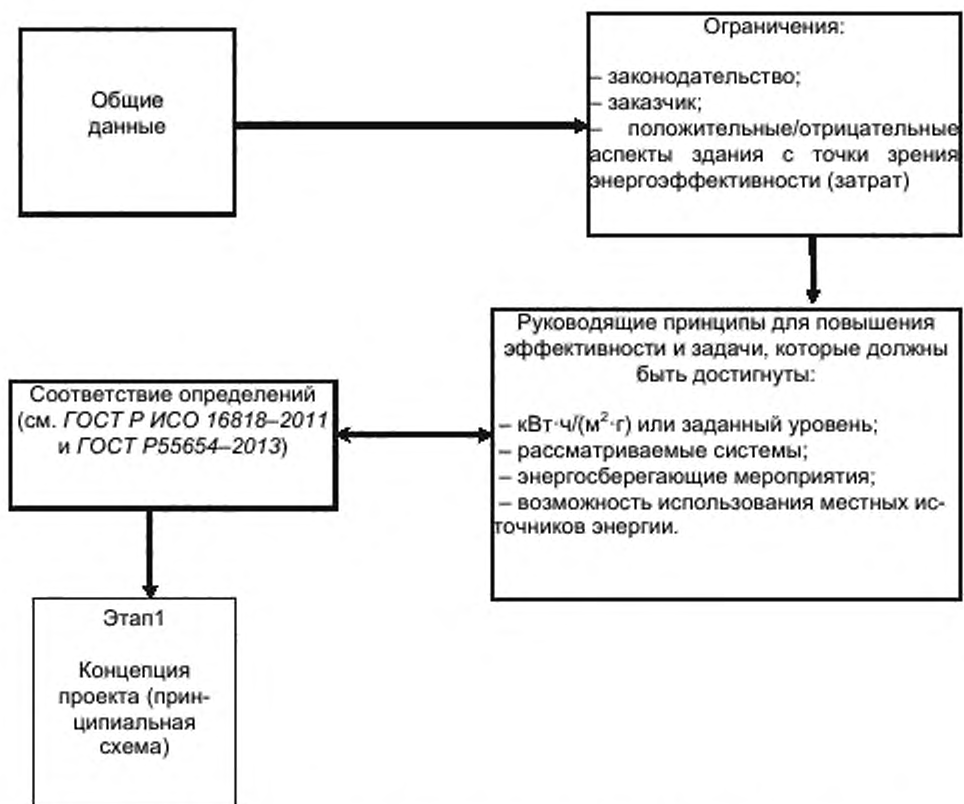
Рисунок А.1 – Блок-схема процесса проектирования энергоэффективности здания
