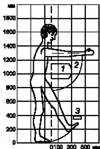
1 — зона размещения часто используемых органов управления (оптимальная зона моторного поля); 2 — зона для размещения часто используемых органов управления (зона легкой досягаемости моторного поля); 3 — органы управления (педали)
