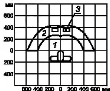
1 — зона размещения часто используемых органов управления (оптимальная зона моторного поля); 2 — зона для размещения часто используемых органов управления (зона легкой досягаемости моторного поля); 3 — органы управления (педали)
