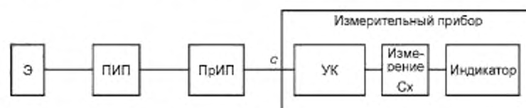
Рисунок Б.2 — Структурная схема, предназначенная для калибровки ИК комплексным методом для индивидуального измерительного прибора
