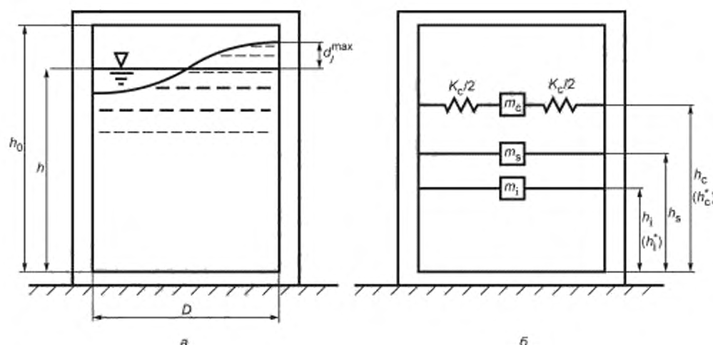
Рисунок 4 — Расчетная модель недеформируемого цилиндрического сосуда с жидкостью, имеющей свободную поверхность
