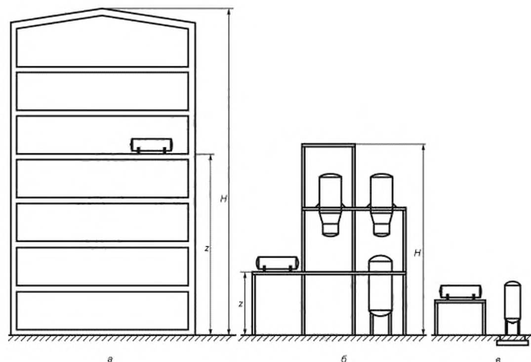
Рисунок 1 — Варианты установки сосуда
