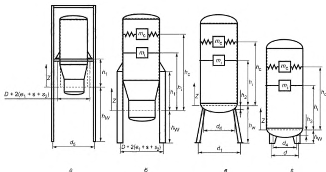
Рисунок 8 — Вертикальный сосуд
