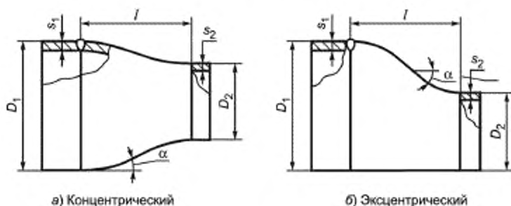
Рисунок 7.2 — Переходы
