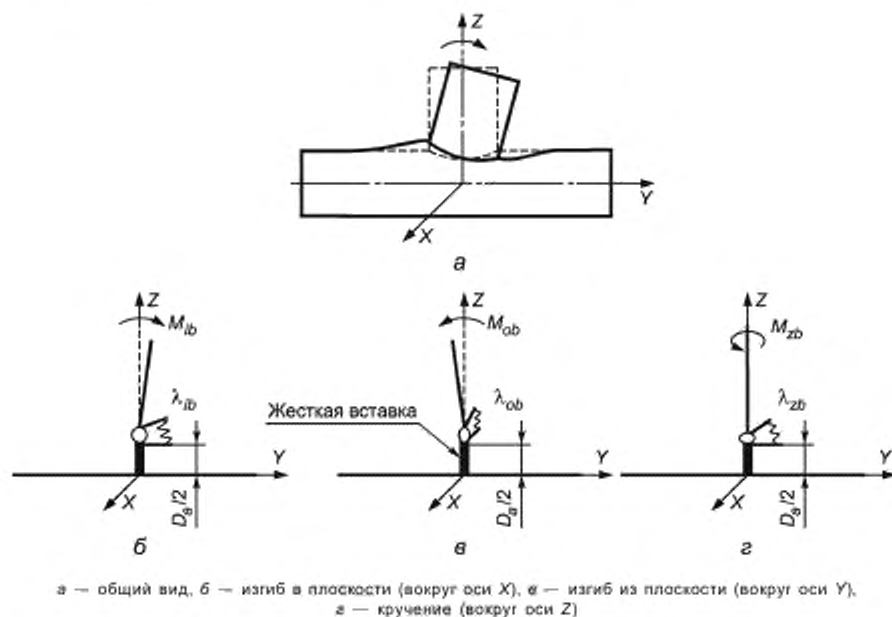
Рисунок A.1 — Расчетная модель тройника (врезки) под нагрузкой со стороны ответвления
