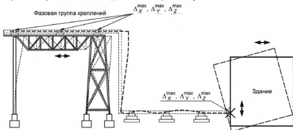
Рисунок 11.3 — Сейсмические смещения креплений
