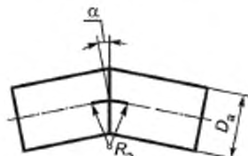
Рисунок 8.8 — Косой стык
