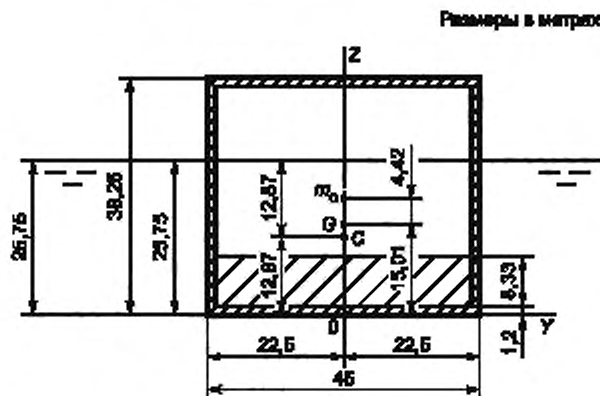
Рисунок К.4 — Поперечное сечение плавящегося объекта по мидель — шпангоуту с основными размерами в м
