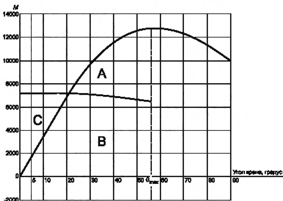
Рисунок 1 — Диаграмма статической остойчивости
