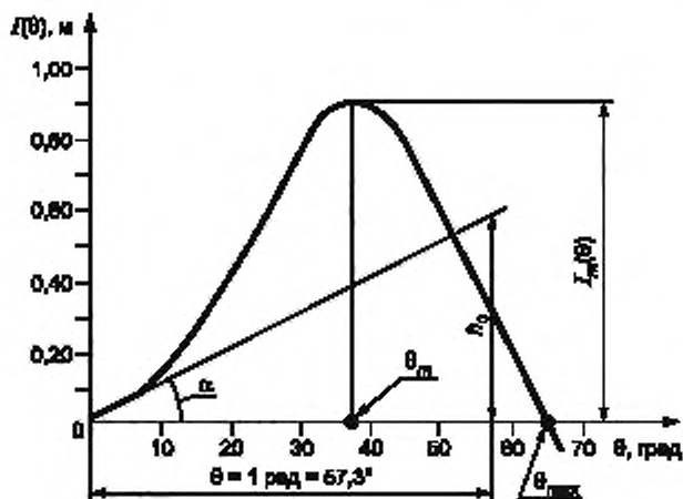
Рисунок К.3 — Диаграмма статической остойчивости
