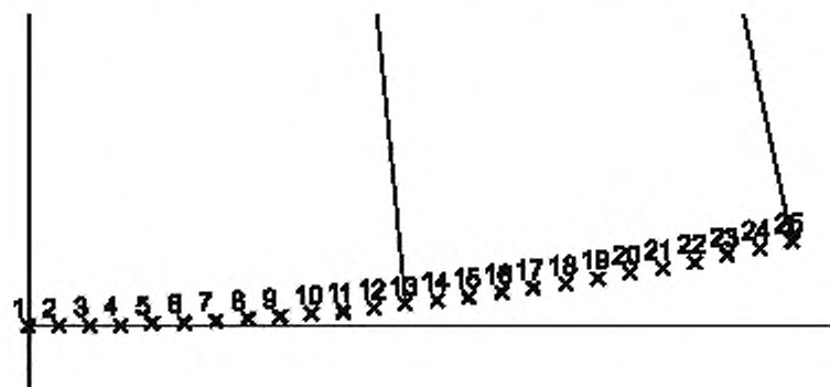
Рисунок К.7 — Укрупненная деталь рисунка К.6 для первых 25 точек перемещения центра величины при кренах плавающего объекта от 0° до 12° с шагом 0,5°
