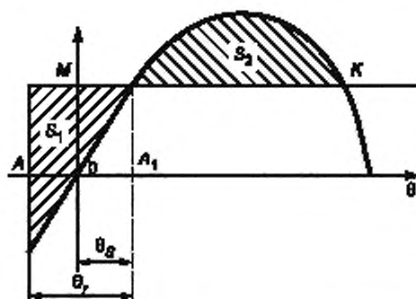
Рисунок 2 — Определение опрокидывающего момента наплавного блока по диаграмме статической устойчивости
