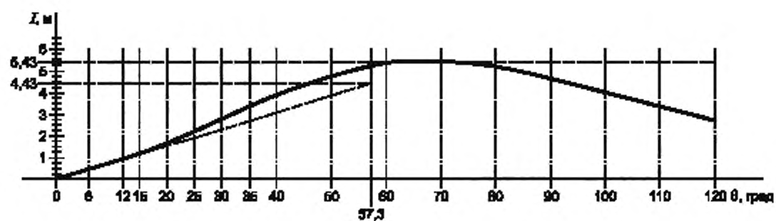
Рисунок К.12 — Диаграмма статической остойчивости
