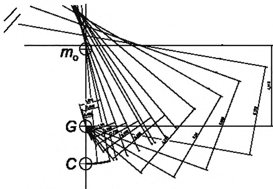
Рисунок К.9 — Измеренные плечи пар сил I(0)_i при кренах от 0° до 90°
