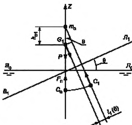
Рисунок К.2 — Плечо статической остойчивости
