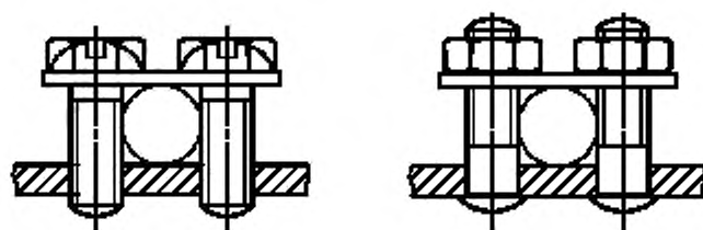
Рисунок 9e — Пластиначные выводы
