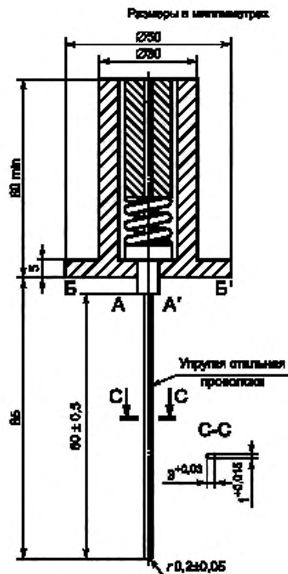
Для проверки калибра к жесткой стальной проволоке прикладывают давящее усилие 20 Н в направлении его оси; характеристики внутренней пружины калибра таковы, что поверхность А-А при прикладывании усилия становится практически вровень с поверхностью В-В.
