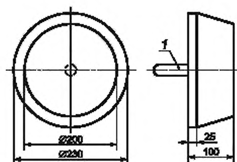
Рисунок Г.5 — Щуп В (большой) для определения застревания головы или шеи пользователя в отверстиях
