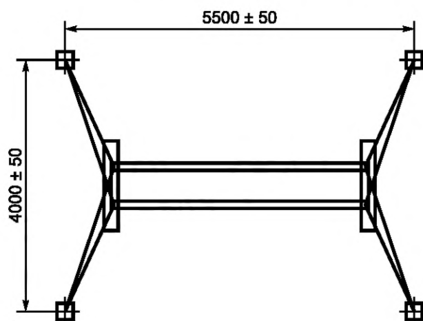
Рисунок 2 — Пример анкерного крепления асимметричных брусьев типа 2
