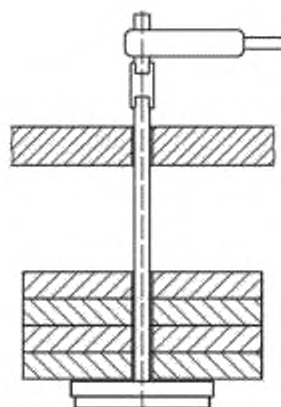
Рисунок 1 — Схема испытательного устройства
