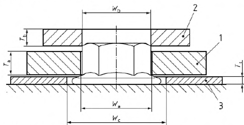
1 — калибр А; 2 — калибр В; 3 — калибр С. W_{A, \text{ макс}} = e_{\text{теор}} ; W_{B, \text{ макс}} = e_{\text{мин}} - 0,01 \text{ мм} ; T_{A, \text{ макс}} = m_{\text{w min}}
