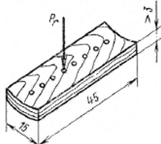
P_r — действие нагрузки в радиальном направлении
