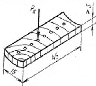
P_a — действие нагрузки вдоль волокон (в торце)
