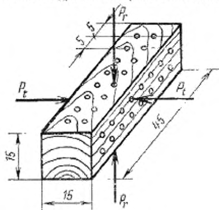
P_r – действие нагрузки в радиальном направлении; P_t – действие нагрузки в тангенциальном направлении
