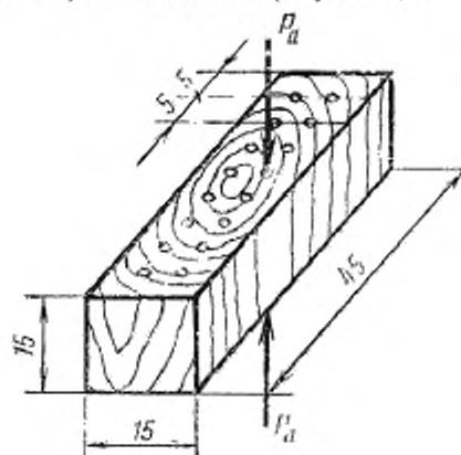
P_a – действие нагрузки вдоль волокон (в торце)
