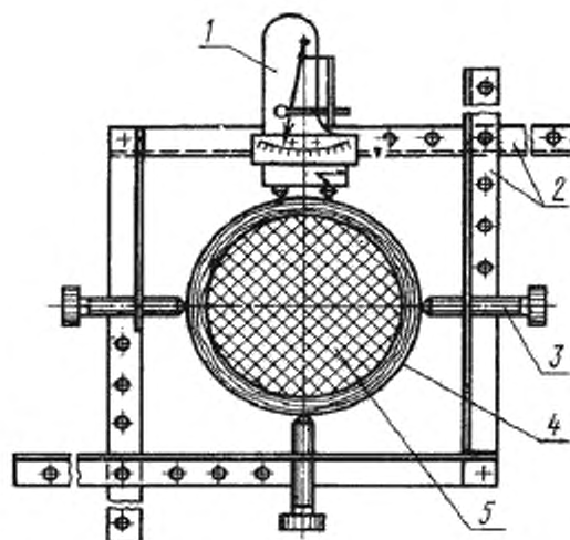
1 – тензометр; 2 – раздвижные планки; 3 – установочные винты; 4 – втулка; 5 – парафин
