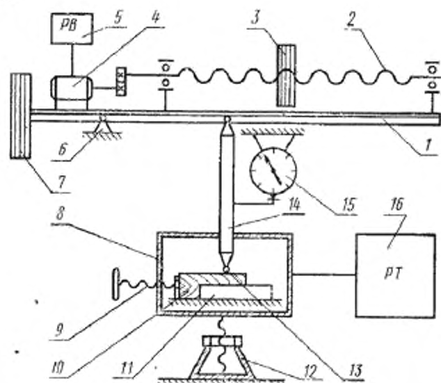
1 – рычаг двухплечный; 2 – винт перемещения груза; 3 – подвижный груз; 4 – реверсивный двигатель с фрикционной передачей; 5 – реле времени; 6 – шарнирная опора рычага; 7 – противовес; 8 – камера; 9 – микрометрический винт перемещения образца; 10 – испытуемый образец; 11 – направляющая образца; 12 – винтовой подъемник; 13 – шарик; 14 – удерживающий шток; 15 – индикатор по ГОСТ 9696; 16 – автоматический регулятор температур
